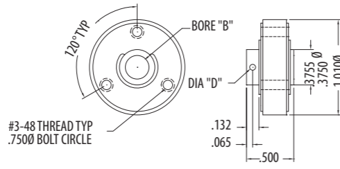
Single Assembly Model HET 3 Tapped Holes
