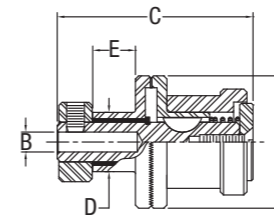
DH CLUTCH - WITH HUB
